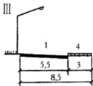
Вулиці та дороги місцевого значення: I – житлові вулиці; II – дороги промислових і комунально-складських зон; проїзди: III – основні; IV – другорядні
