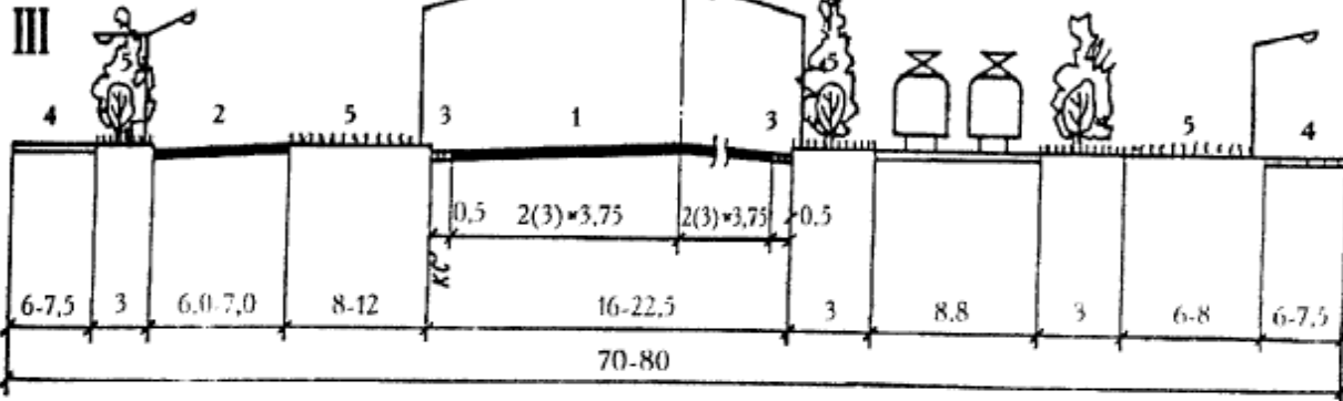
Магістральні вулиці загальноміського значення: I – безперервного руху; II, III – регульованого руху
